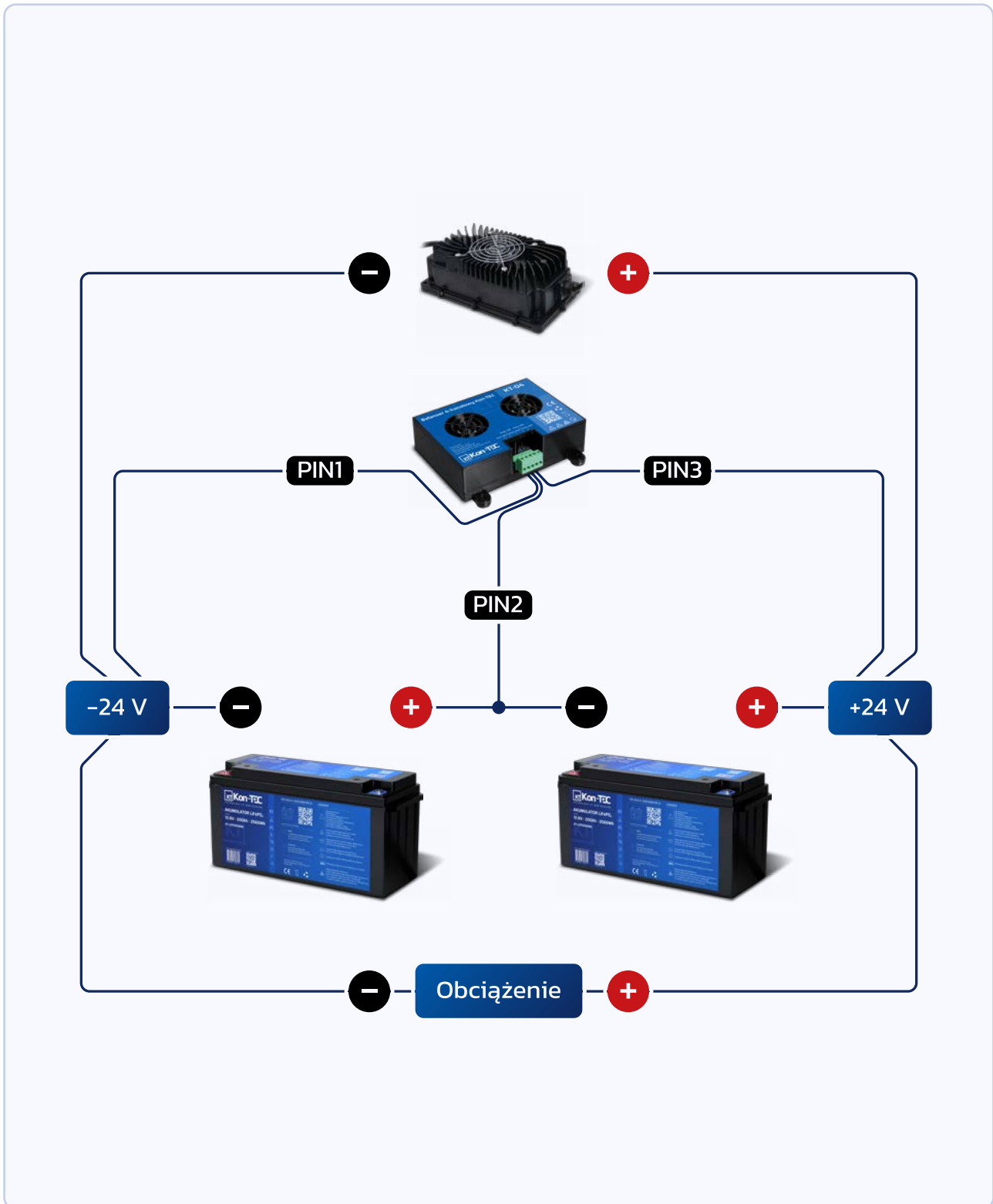
Rys. 4. Schemat połączenia szeregowego i balansera (24 V).
