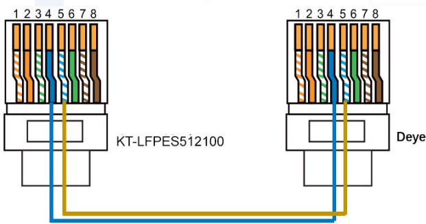
Połączenie z Deye Inwerter hybrydowy
