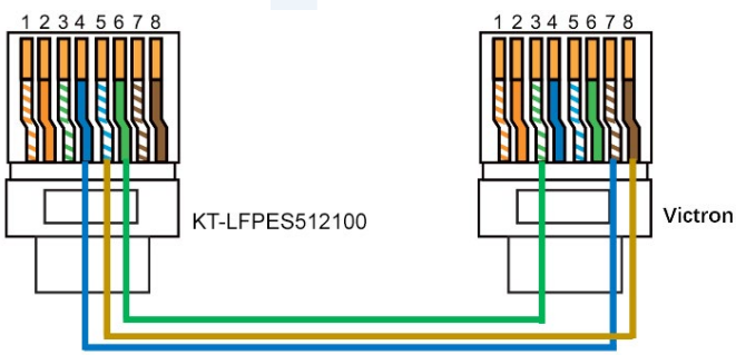
Połączenie z Victron GX Inwerter/ładowarka
