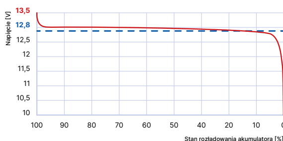
Rys. 1. Spadek napięcia akumulatora, rozładowanie 1C
