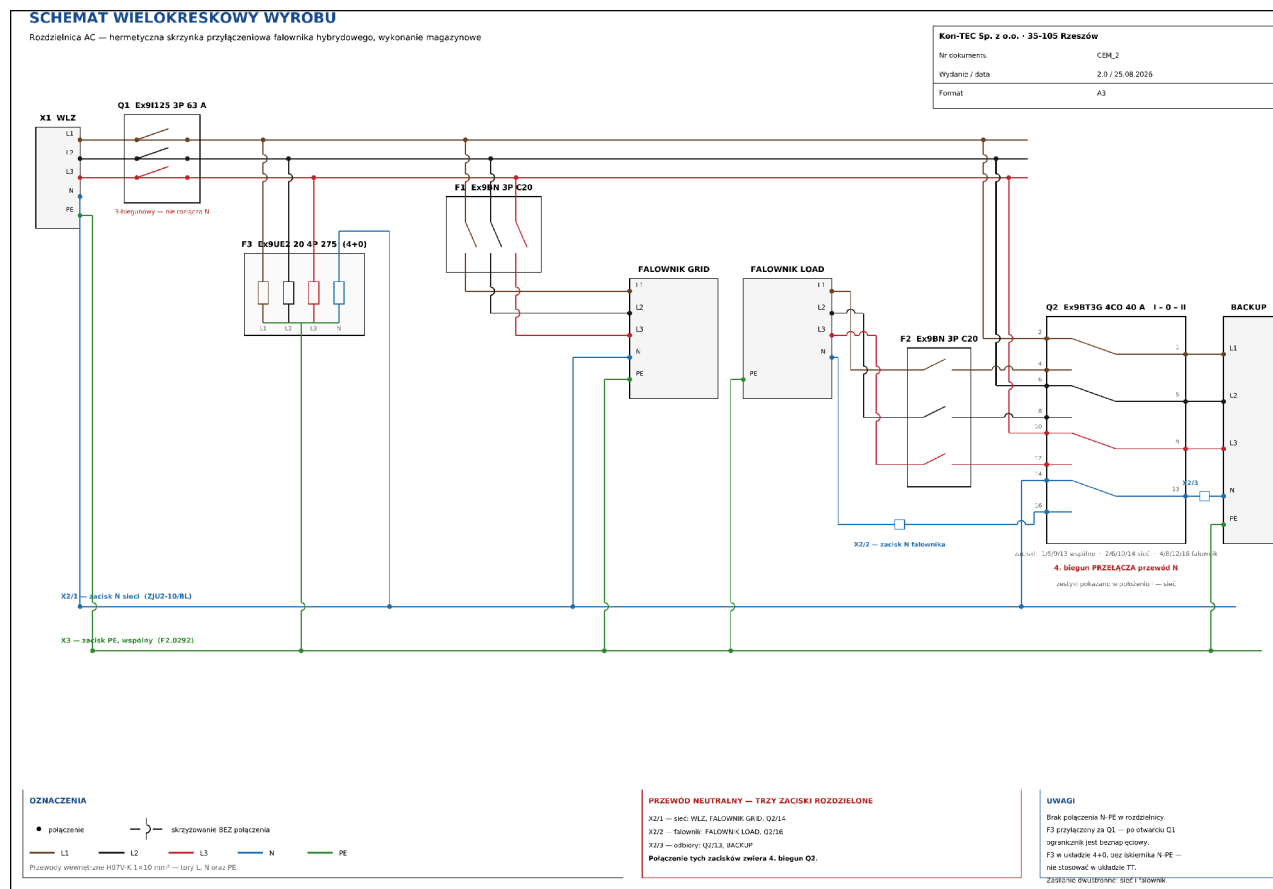
Rys. 1. Schemat wielokreskowy rozdzielnic — wykonanie magazynowe. Odzworowanie dokumentu CEM_2, wyd. 2.0 z 25.08.2026; oryginał w formacie A3.
