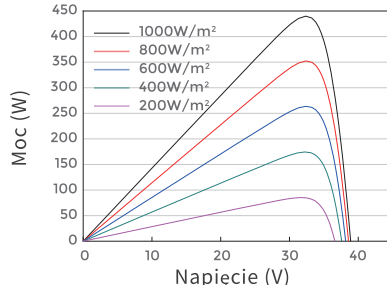
Krzywa moc – napięcie JAM54D41-440/LB
