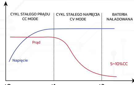
Rys.1. Metoda ładowania ładowarkami Kon-TEC z serii DL.
