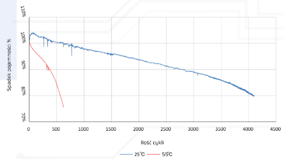
Rys. 2 Żywotność w różnych temperaturach, 1C
