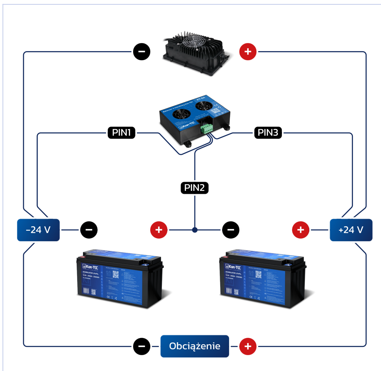
Rys. 4. Schemat połączenia szeregowego i balansera (24 V).
