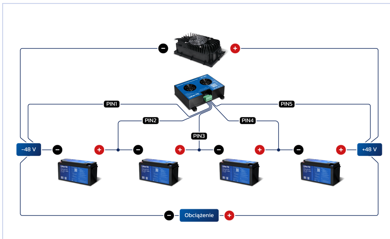
Rys. 6. Schemat połączenia szeregowego i balansera (48 V).
