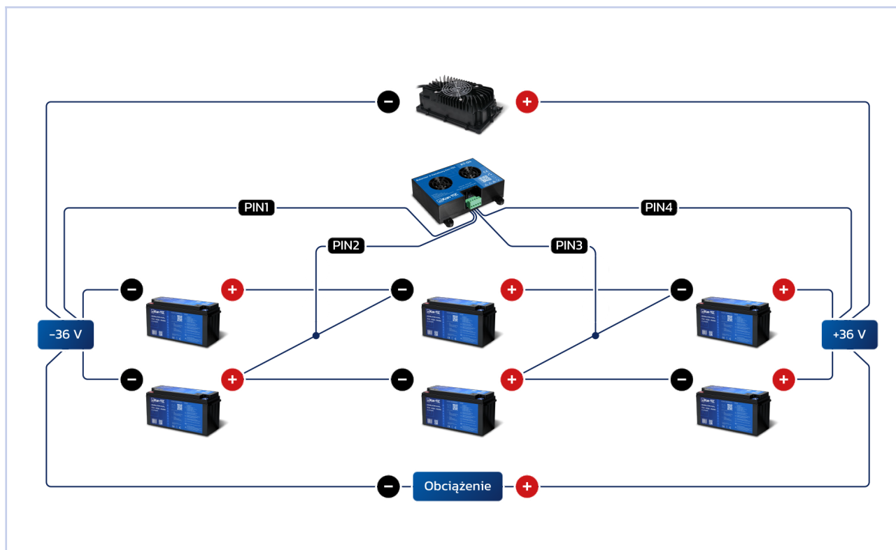
Rys. 8. Schemat połączenia szeregowo-równoległego i balansera (36 V).
