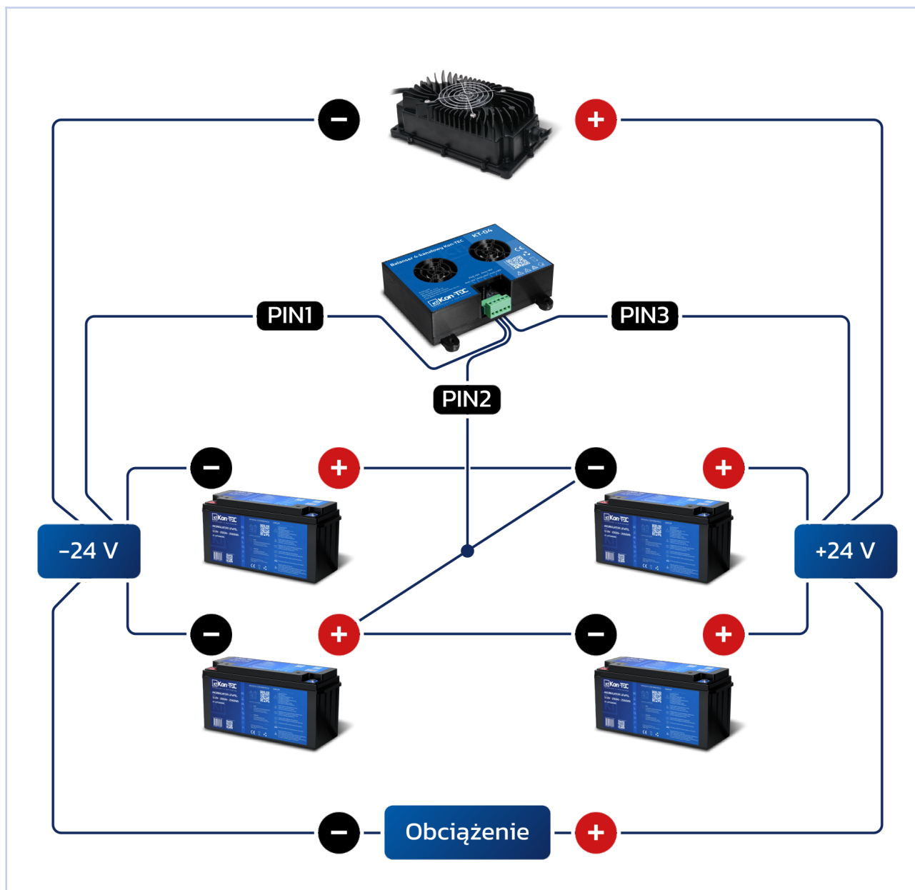
Rys. 7. Schemat połączenia szeregowo-równoległego i balansera (24 V).
