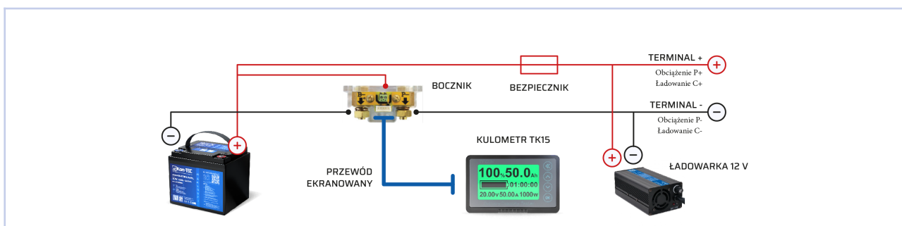
Rys. 1. Schemat podłączenia pojedynczego akumulatora.
