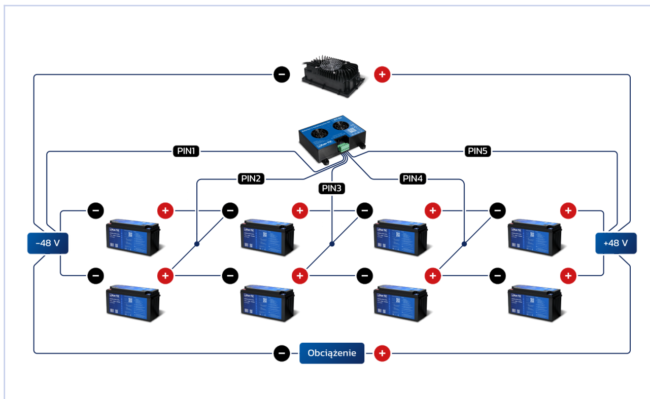
Rys. 9. Schemat połączenia szeregowo-równoległego i balansera (48 V).
