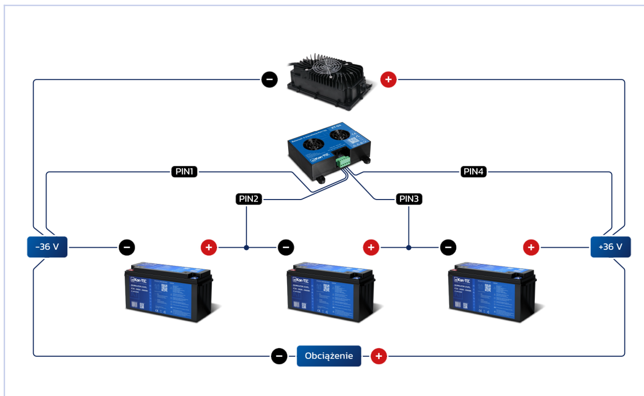
Rys. 5. Schemat połączenia szeregowego i balansera (36 V).
