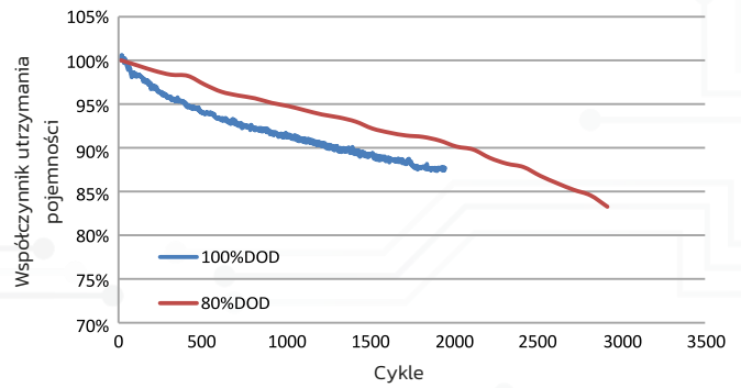
Krzywa cyklu życia przy różnych stopniach rozładowania (DOD) 0,5C @RT
