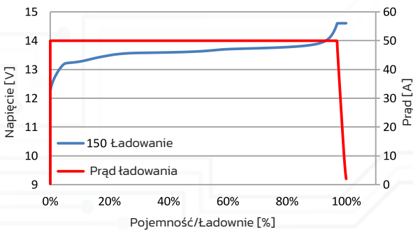
Charakterystyka ładowania 0,5C @RT
