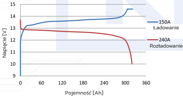
Krzywa pojemności ładowania-rozładowania @RT
