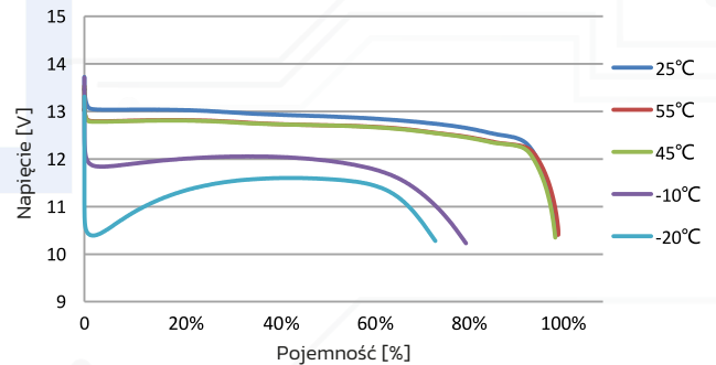
Krzywe rozładowania przy różnych temperaturach
