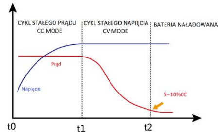
Rys.1. Metoda ładowania ładowarkami Kon-TEC z serii DL
