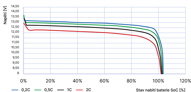
Obr. 8. Napětí baterie při vybíjení při různých proudech
